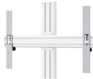
VESA-Bügel 200/400 mm 9108* (Set inkl. Neigungseinstellung)
